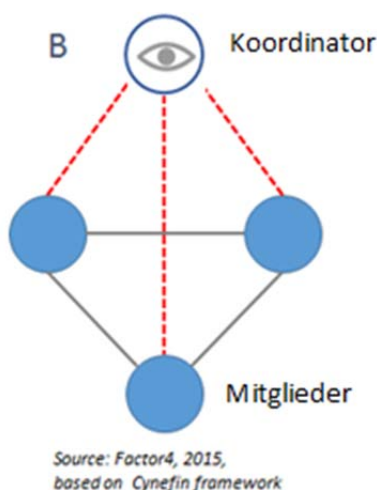
Abbildung 1: Komplexer SPIN
